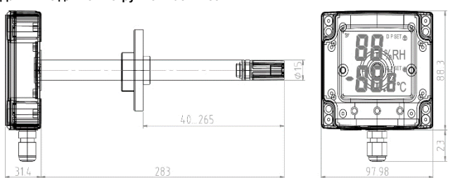
Размеры датчика, мм
