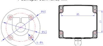
Установочные размеры, мм
